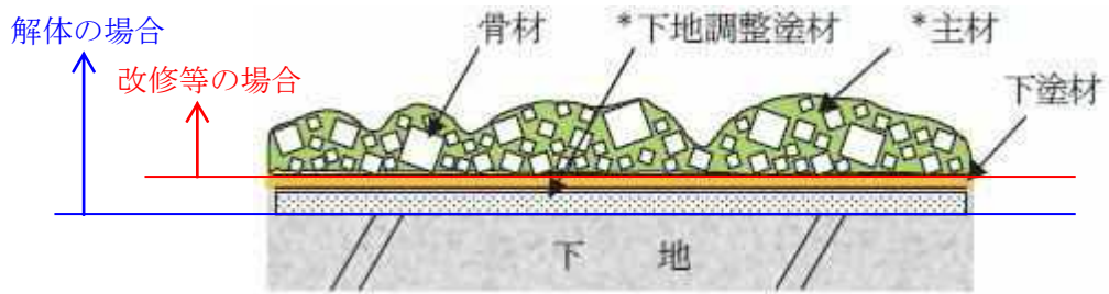
【厚付け仕上塗材（上塗材なし）：吹放し模様の例】
